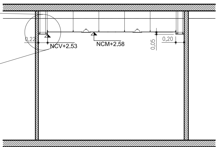
CORTE B-B
