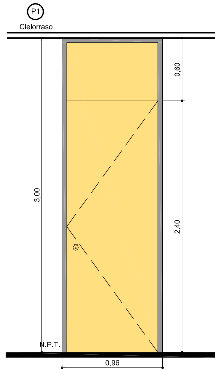
Puerta placa enchapada en madera maple Marco Modena hombro recto en aluminio anodizado natural Cerradura Tipo Pomo Meroni Forma Nº 13 NA
