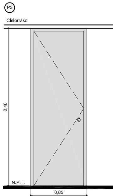
Puerta placa enchapada en melamina color blanco Marco en madera pintada Cerradura Tipo Pomo Meroni Forma Nº 13 NA Cierrapuerta aéreo apto 50 kg. Terminación Aluminio anodizado natural
