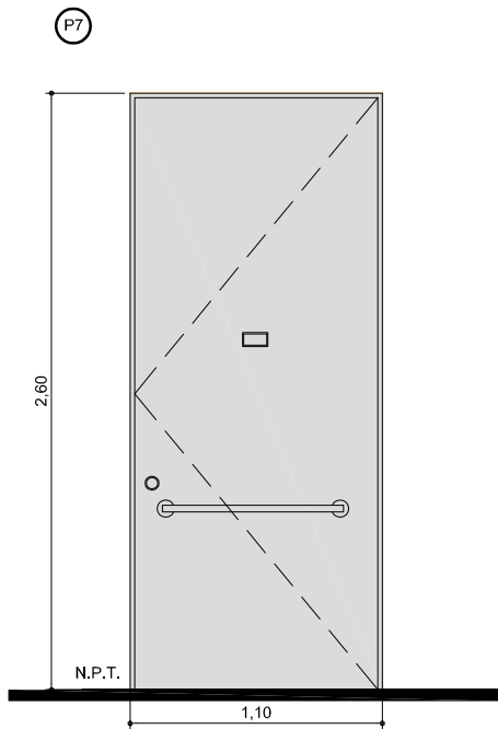
Hoja y marco en chapa doblada Pintada s/especificaciones Barral antipánico marca Jaque con cerradura de seguridad y mirilla Cierrapuerta aéreo apto 60 kg. Terminación Aluminio anodizado natural
