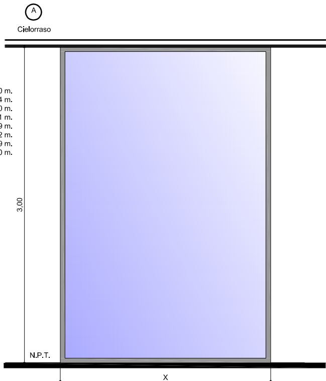
Vidrio templado e= 10 mm. - Junta a tope siliconada Perfil Modena hombro recto de aluminio anodizado natural
