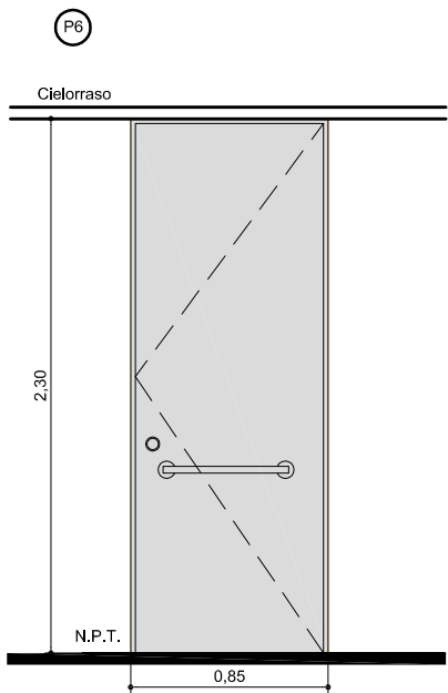
Hoja en chapa inyectada F60 Marco en chapa doblada Pintada s/especificaciones Barral Antipánico marca Jaque con cerradura de seguridad y cierra puerta aéreo apto 60 kg. Terminación Aluminio anodizado natural
