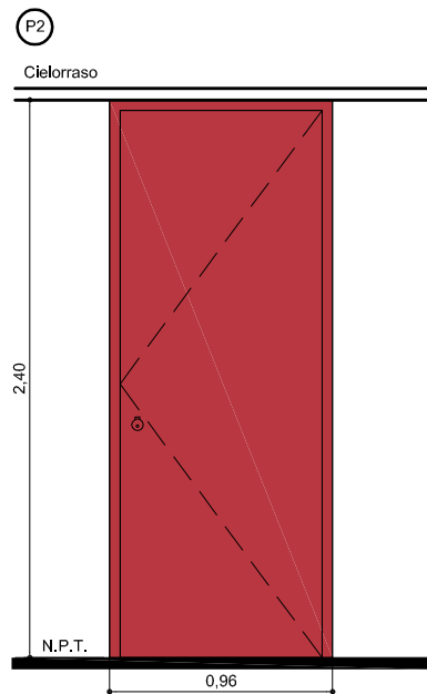
Puerta placa pintada color institucional Marco en madera pintado color institucional Cerradura Tipo Pomo Meroni Forma Nº 13 NA
