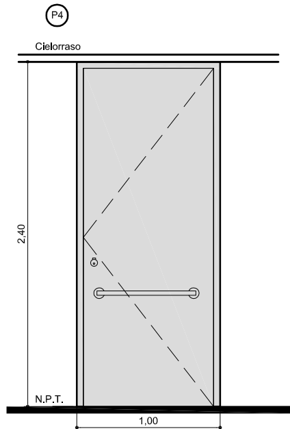
Puerta placa enchapada en melamina color blanco Marco en madera pintada Cerradura Tipo Pomo Meroni Forma Nº 13 NA Barral horizontal para discapacitados
