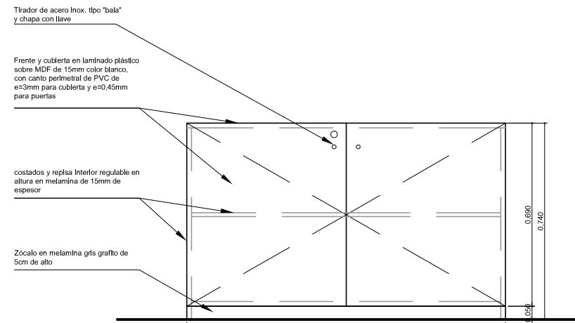
FRENTE mueble especial 6 - Recepción Mueble de archivo Esc:1/20
