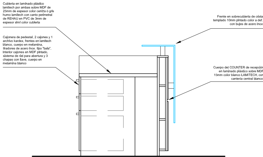
CORTE mueble especial 6 - Recepción Esc:1/20
