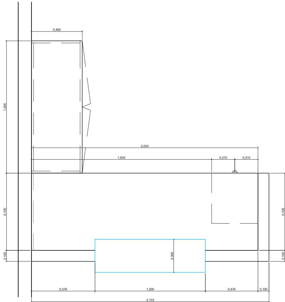
PLANTA mueble especial 6 - Recepción Esc:1/20
