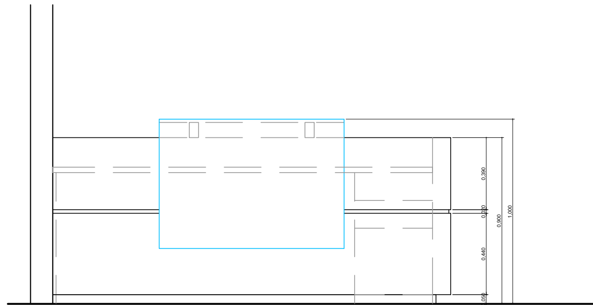
FRENTE mueble especial 6 - Recepción Esc:1/20
