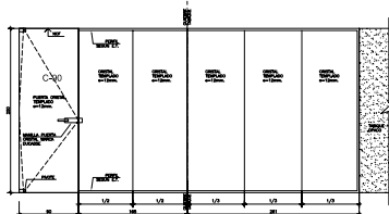
ELEVACION TABIQUE CRISTAL N° 6
