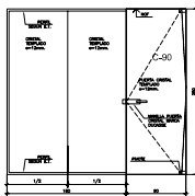
ELEVACION TABIQUE CRISTAL N° 7
