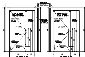
ELEVACION TABIQUE CRISTAL N° 1
