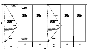
ELEVACION TABIQUE CRISTAL N° 4
