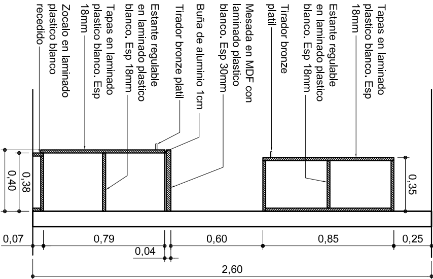
CORTE B-B
