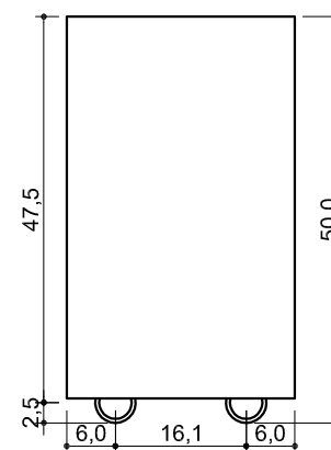
VISTA 01 MESA DE APOYO - ESTAR ESC. 1:10
