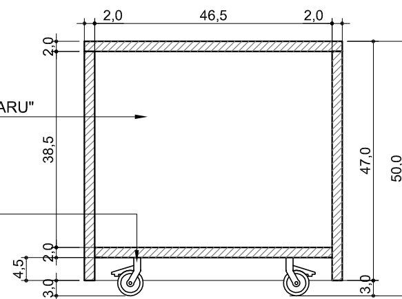
CORTE AA' MESA DE APOYO - ESTAR ESC. 1:10
