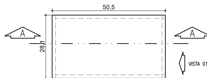
PLANTA MESA DE APOYO - ESTAR ESC. 1:10
