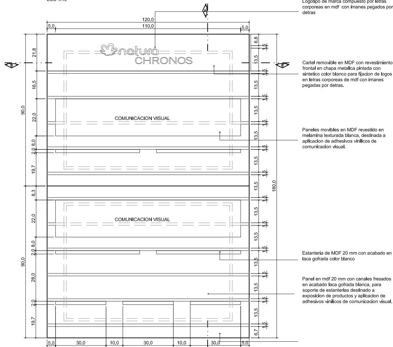
CORTE BB PANEL EXPOSITOR CHRONOS ESC 1:10
