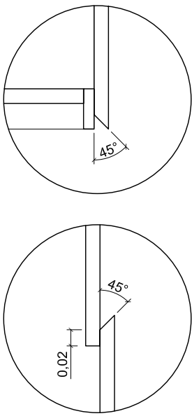
DETALLES TIRADOR TIPO CAVA ESC 1/5
