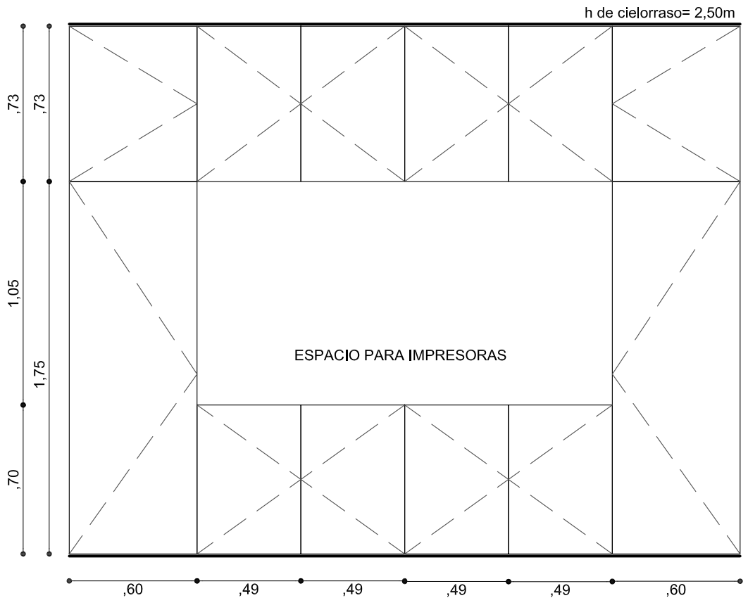
VISTA FRENTE
