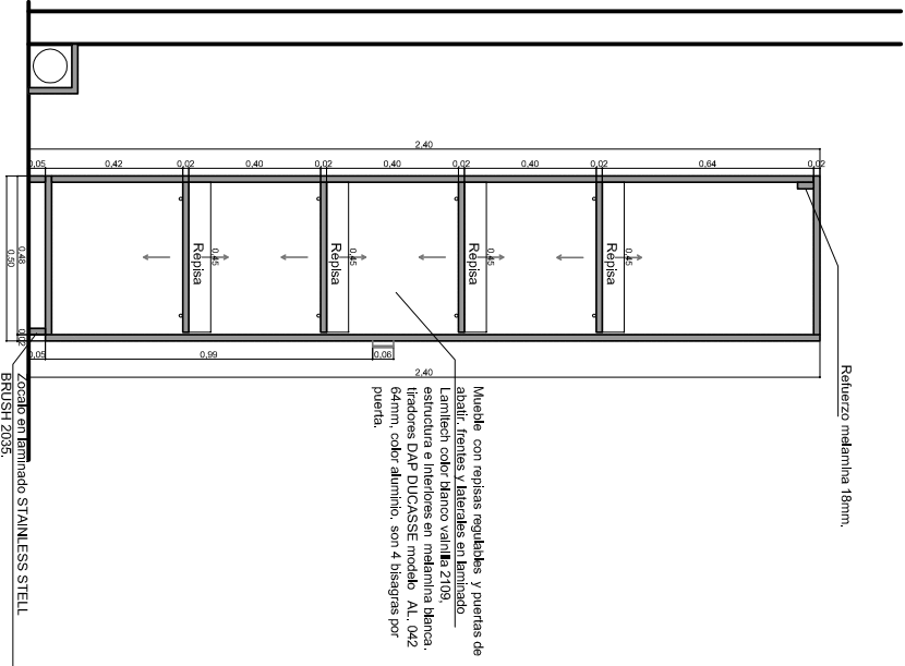
corte elevacion 2 esc 1/25
