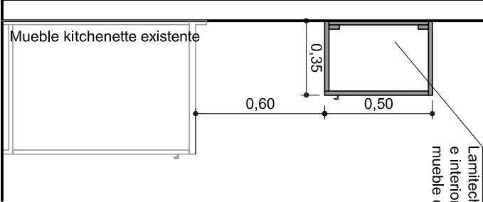
corte elevacion 1 esc 1/25
