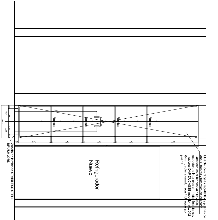
elevacion 2 esc 1/25
