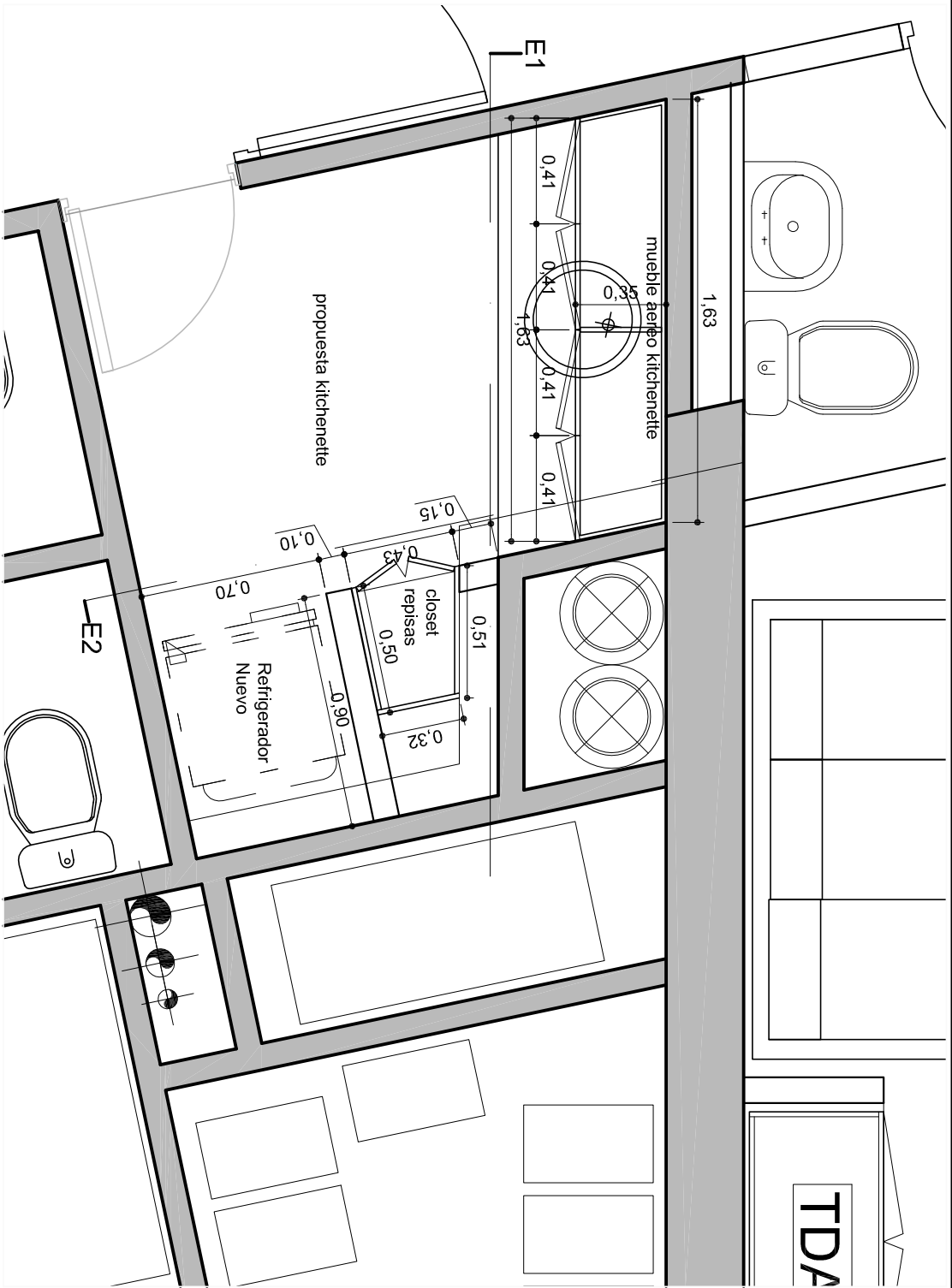
Layout propuesta Kitchenette esc 1/25
