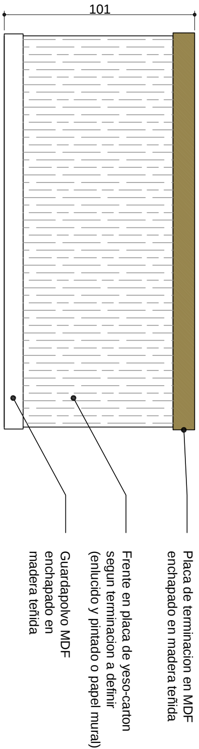
Elevacion frontal
