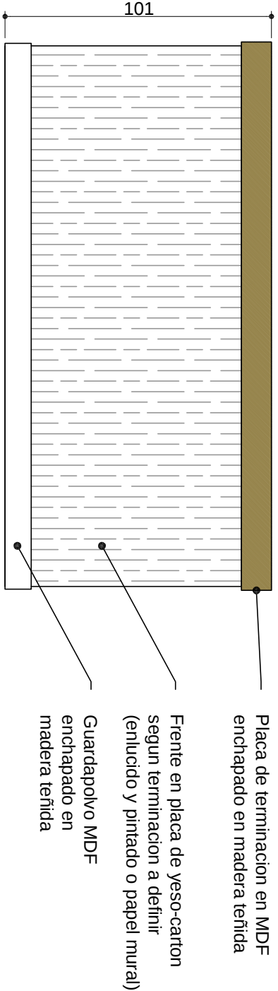
Elevacion frontal
