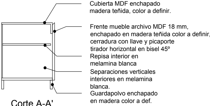
Corte A-A'
