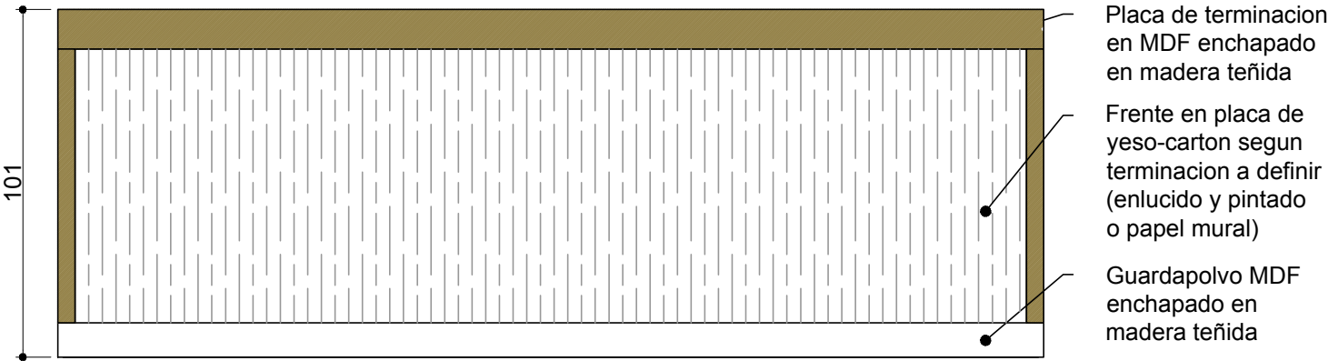
Elevacion frontal
