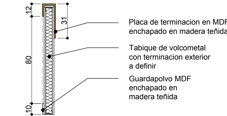
Corte A-A
