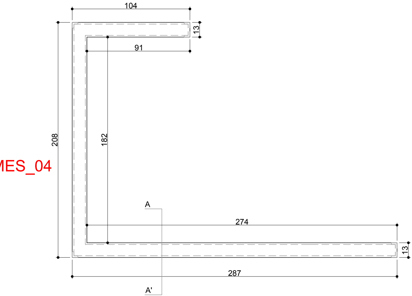
Planta muro apoyo asistente 1
