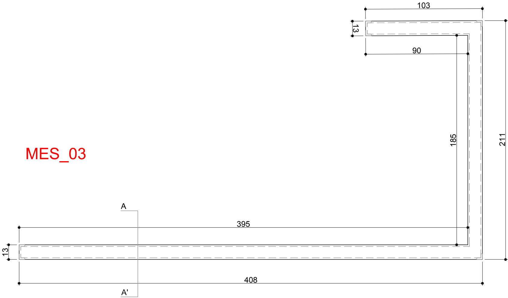
Planta muro apoyo asistente 1
