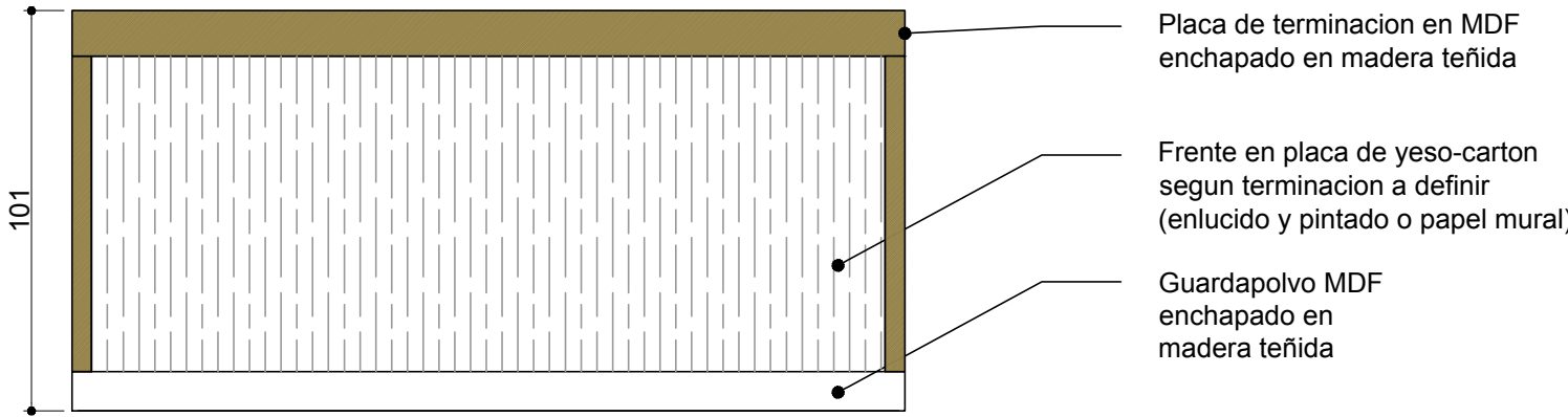
Elevacion frontal
