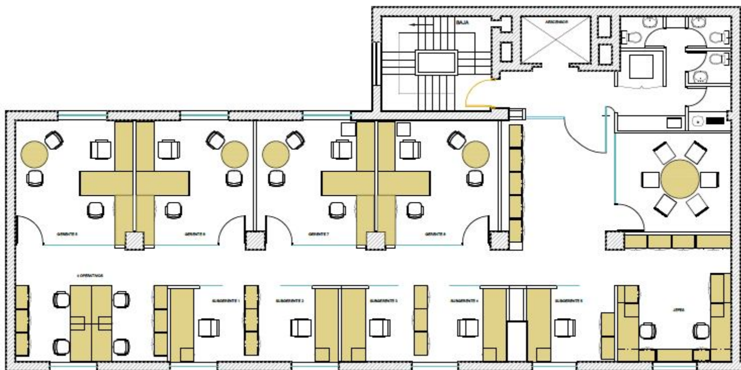
PLANTA 4TO PISO ESTADO
