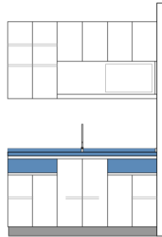
ELEVACION FRONTAL ME 5 ESC. 1:25
