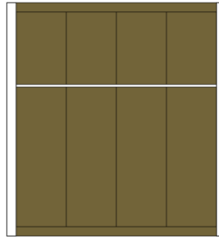
ELEVACION FRONTAL ME 1 ESC. 1:25
