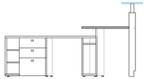
CORTE A-A ME 3 ESC. 1:25
