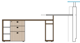
CORTE B-B ME 3 ESC. 1:25
