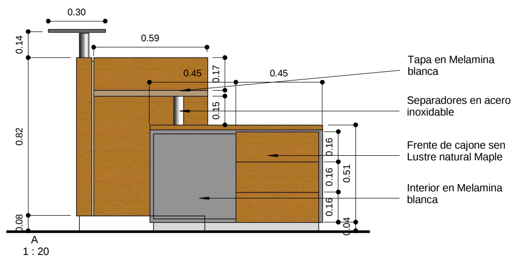
Vista - 1 1:20
