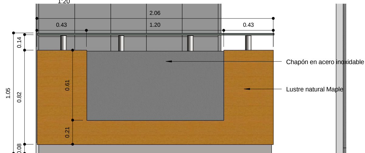
Vista Frontal 1:20
