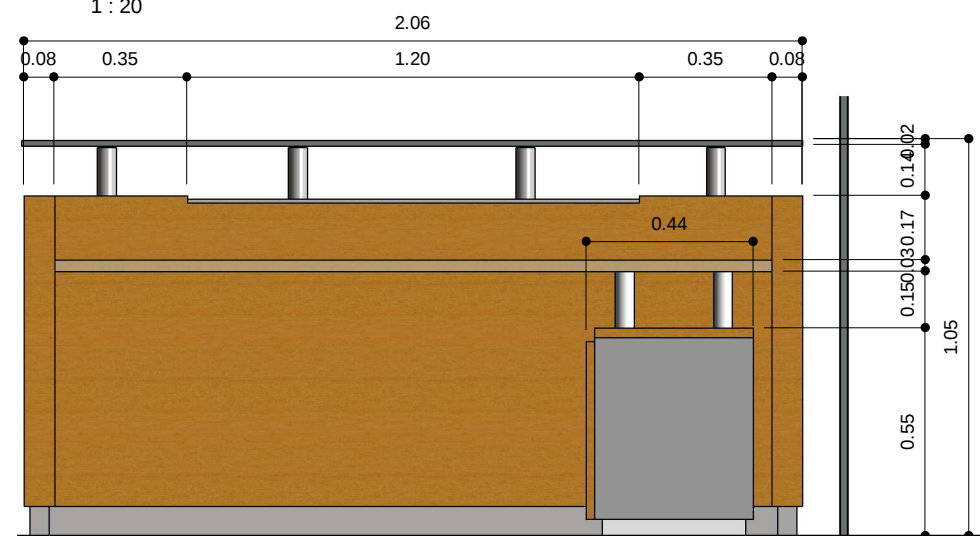
Vista Contrafrente 1:20
