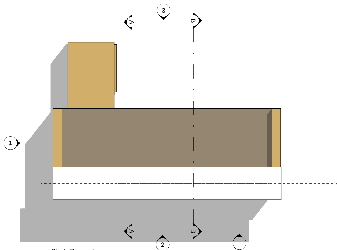
Planta Recepción 1:20
