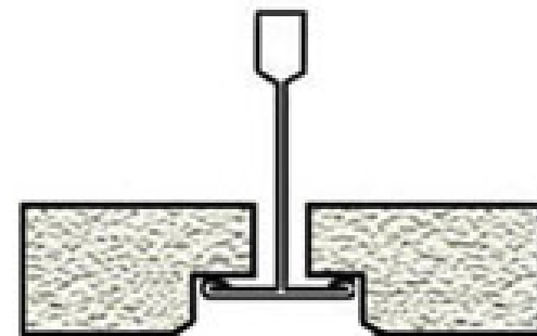
Cielo Modular modelo Existente 61x61cm de fibra mineral canto rebajado.
