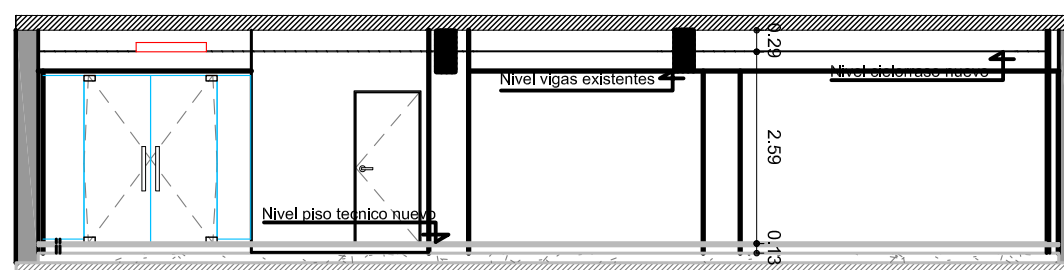
CORTE TRANSVERSAL
