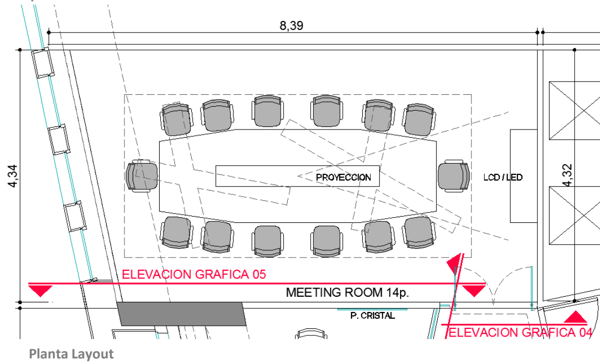
Muro de cristal con film IMPRESO. Sala de reuniones 14 personas.
