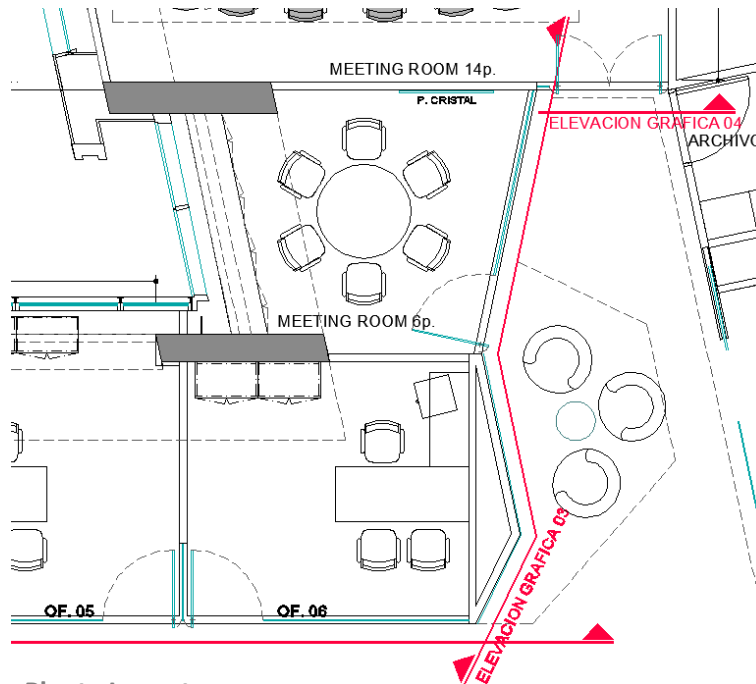
Planta Layout
