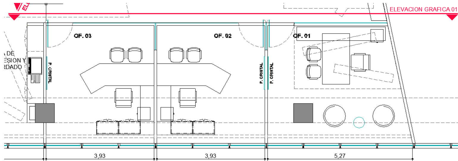
Planta Layout
