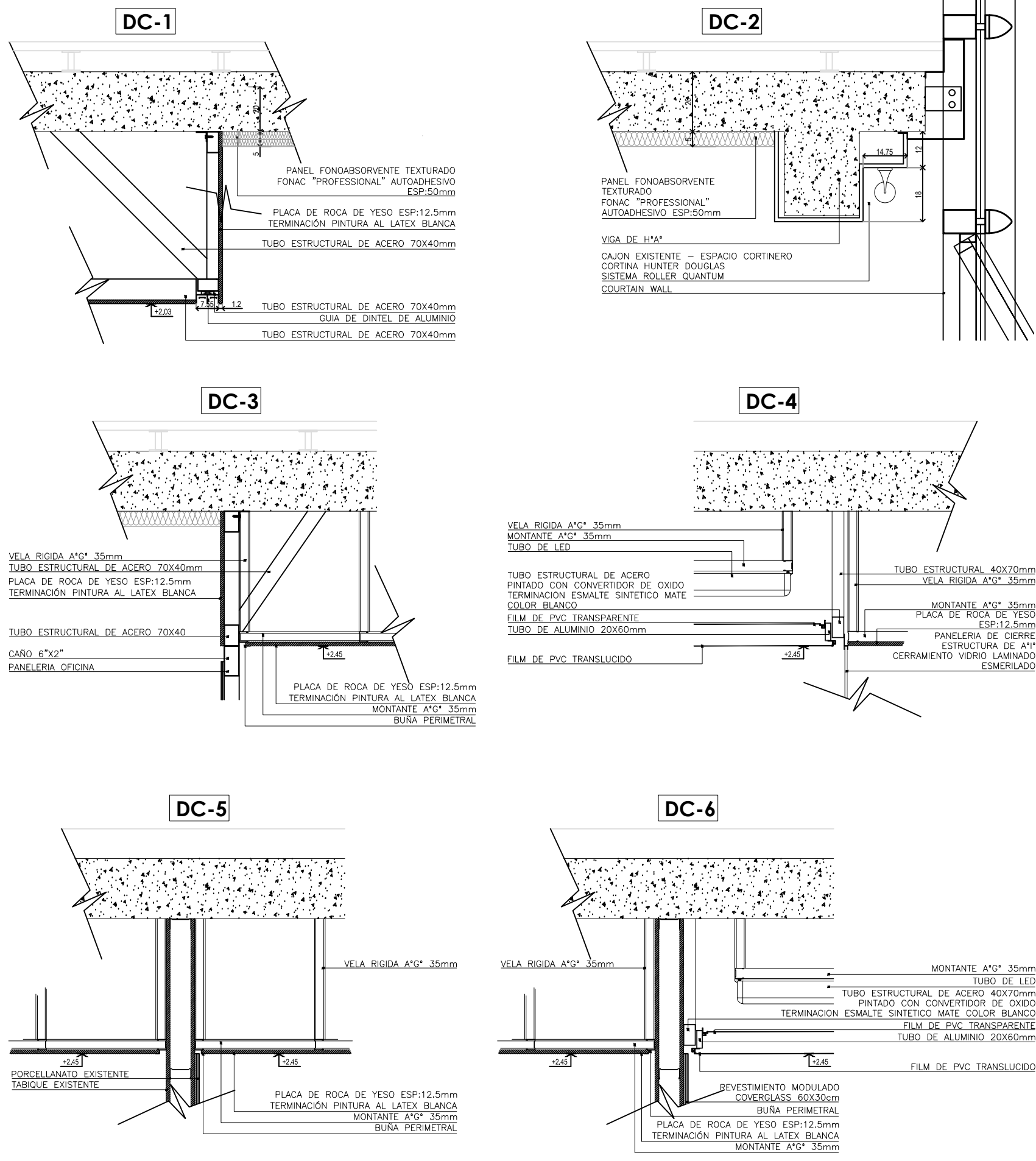
DETALLES CIELORRASOS ESC. 1:15
