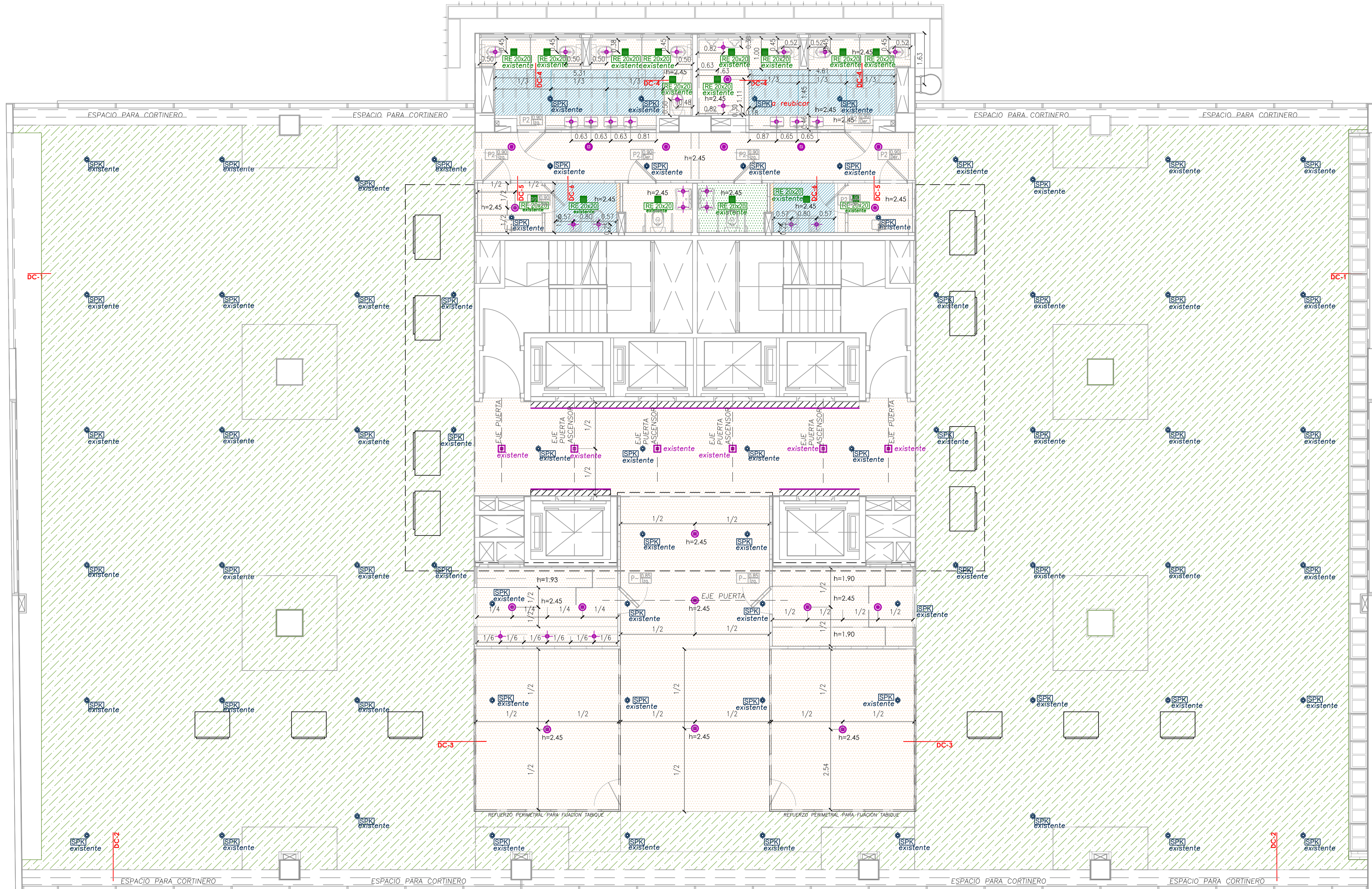
5° PISO - PLANTA CIELORRASOS ESC. 1:75
