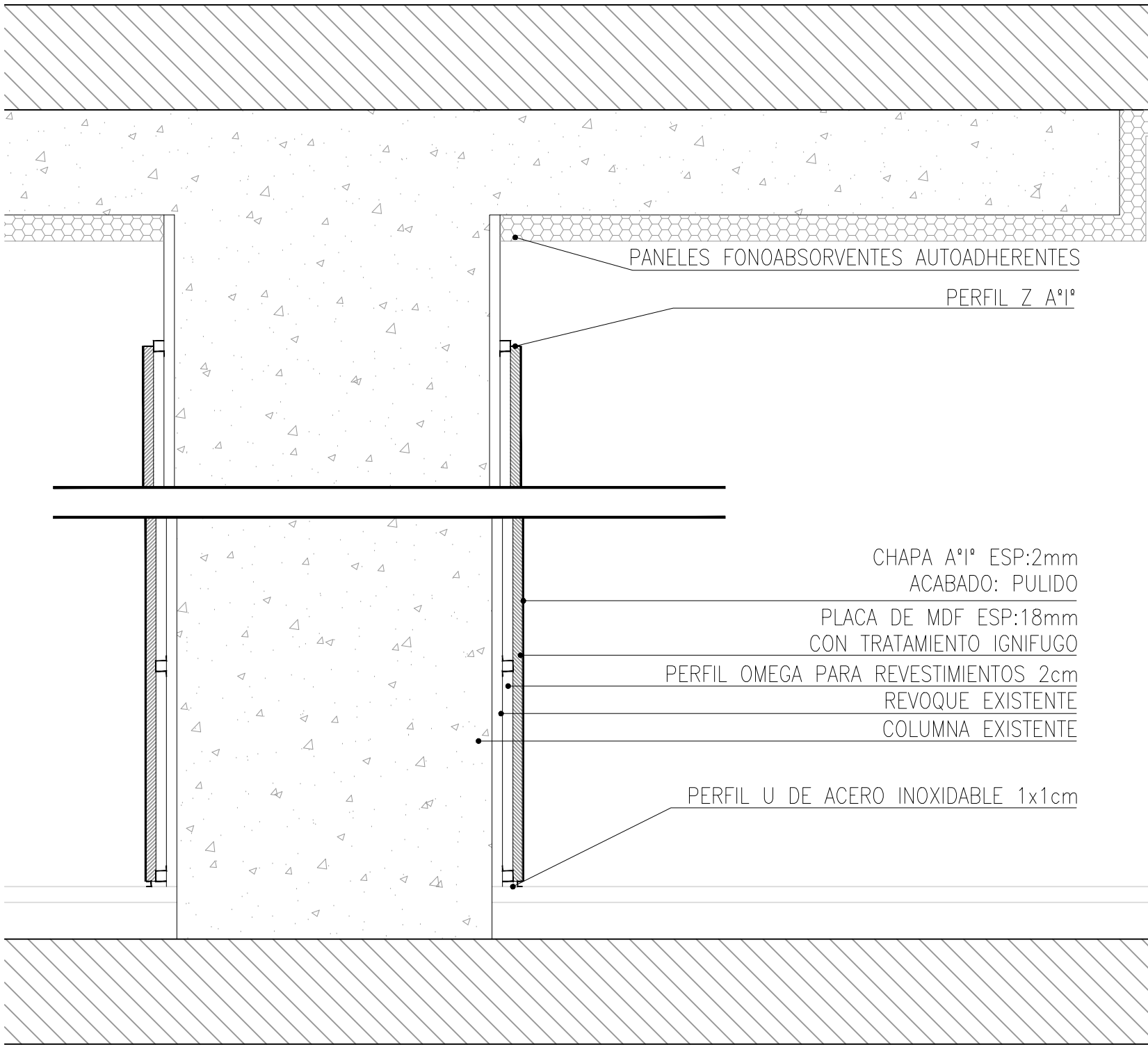
C3-CORTE ESC. 1:10
