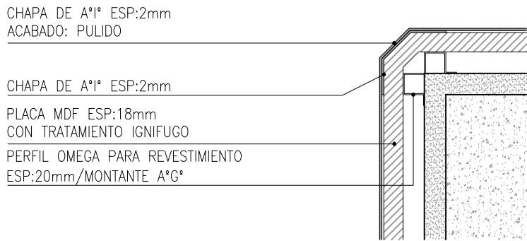
DETALLE ESQUINA 2 ESC. 1:5
