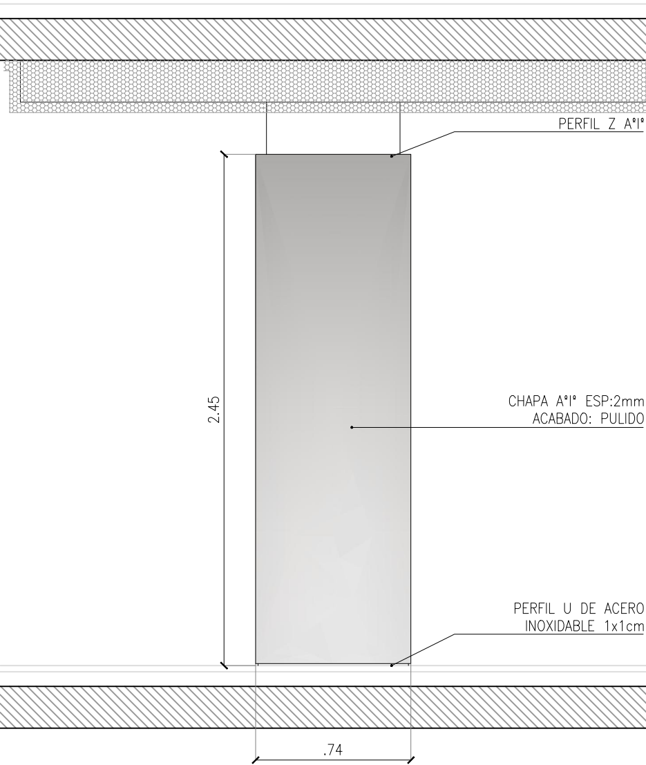
C3-VISTA 1 ESC. 1:25
