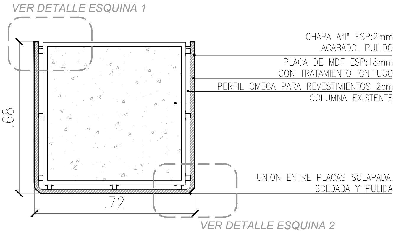
C3-PLANTA ESC. 1:10
