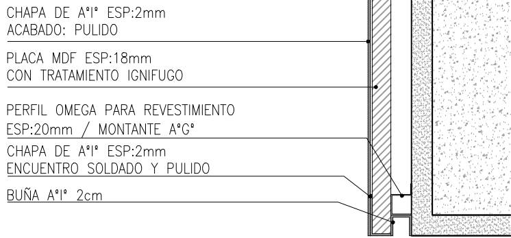
DETALLE ESQUINA 1 ESC. 1:5
