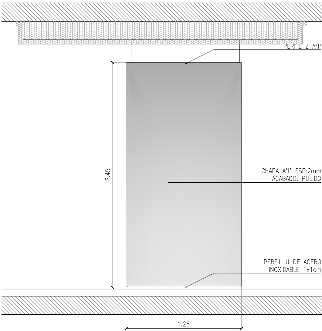
C4-VISTA 1 ESC. 1:25
