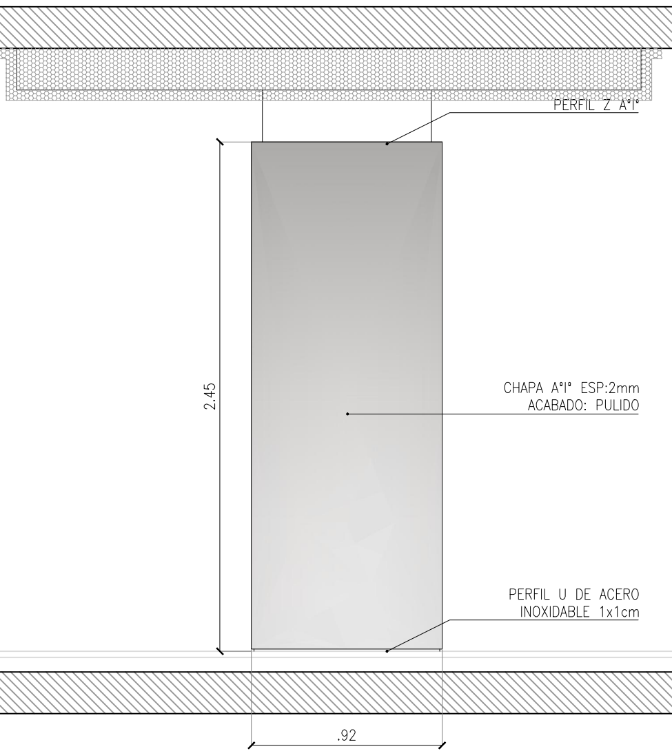
C4-VISTA2 ESC. 1:25
