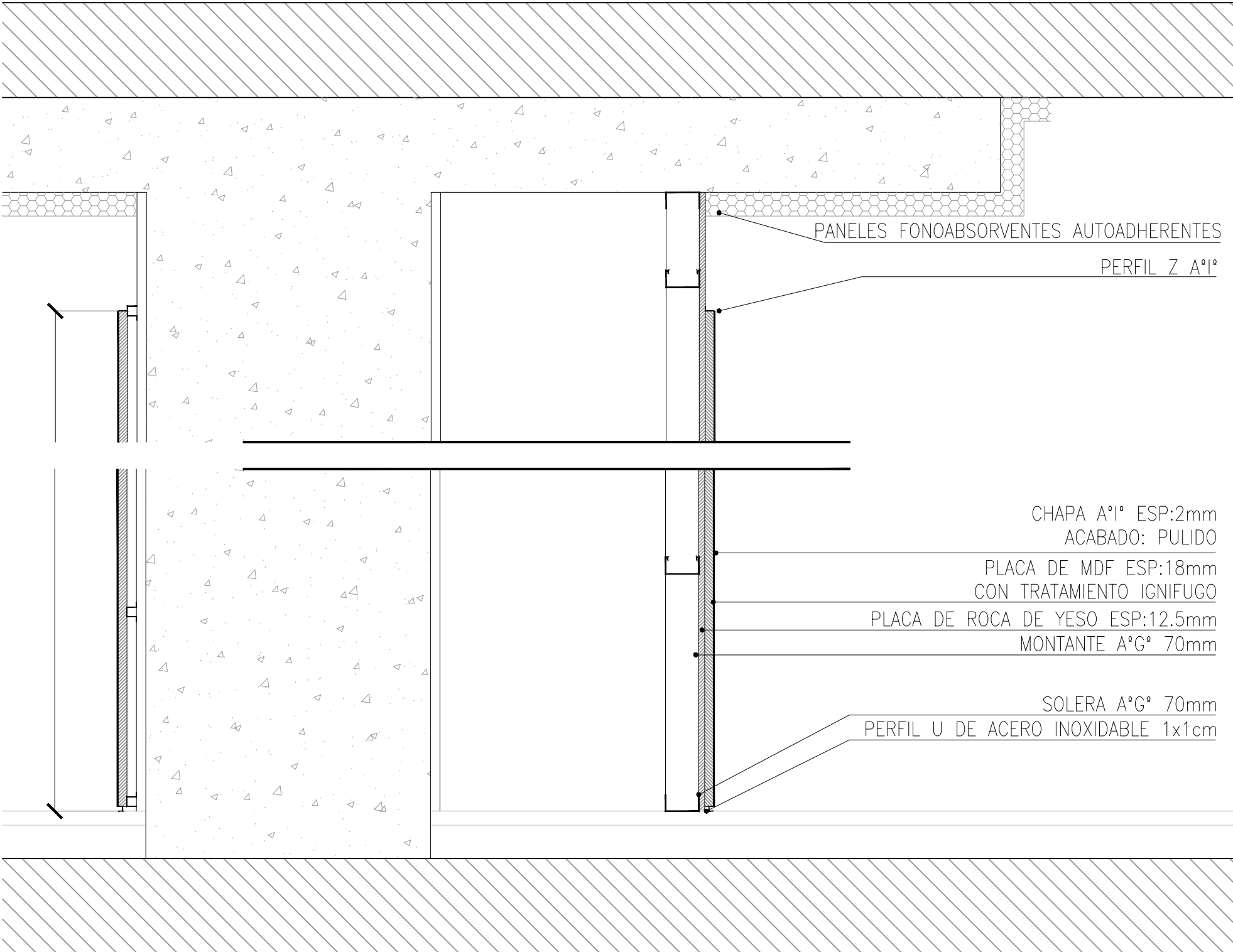
C4-CORTE ESC. 1:10
