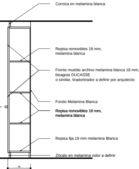
CORTE A-A'
