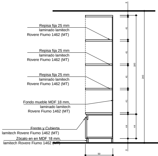
CORTE B-B'
