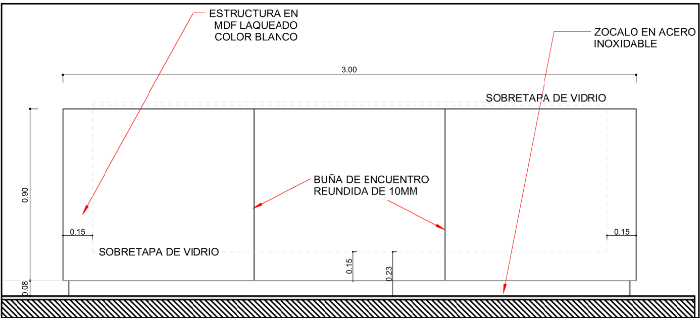
VISTA FRENTE
