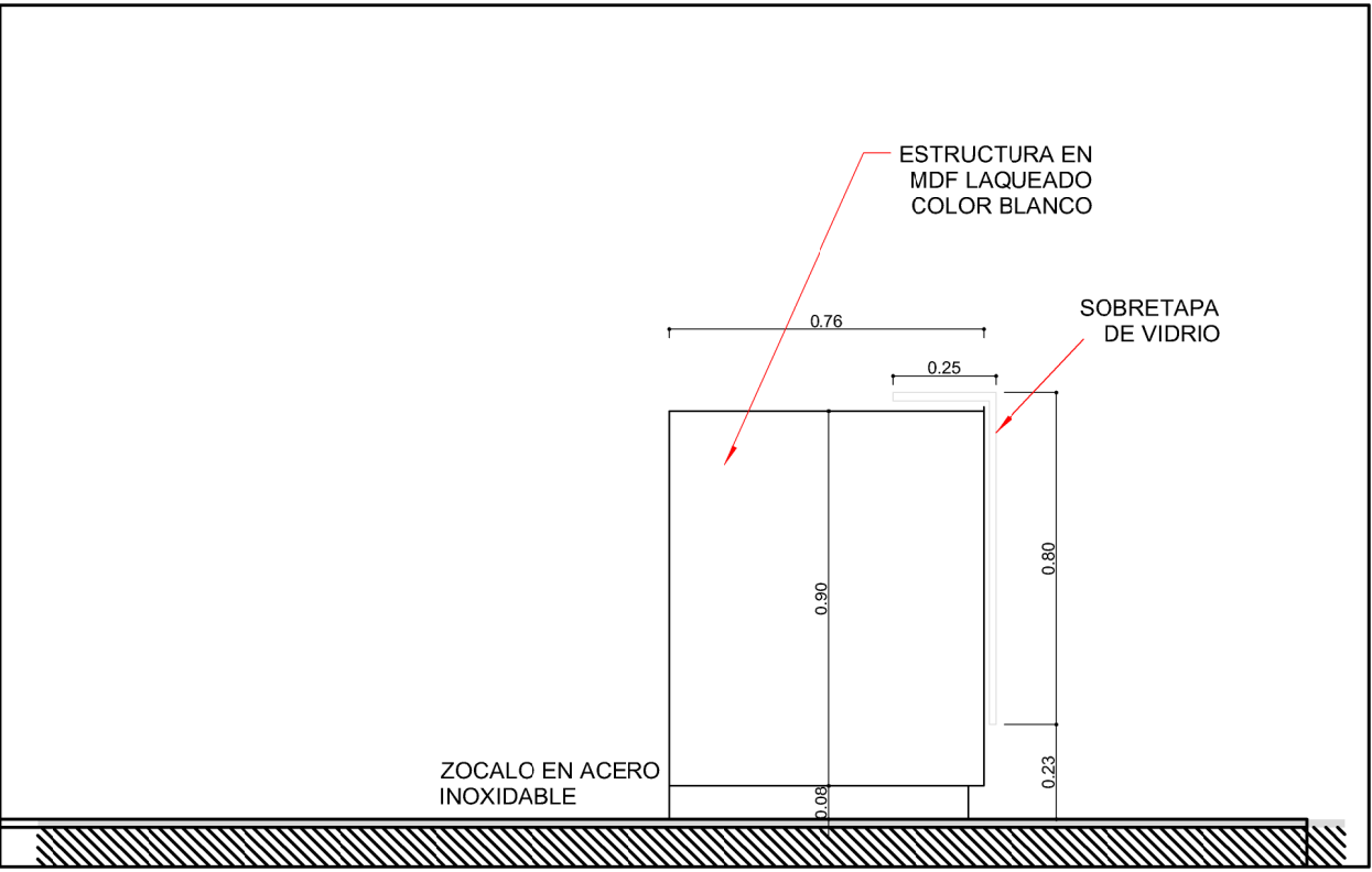
VISTA LATERAL
