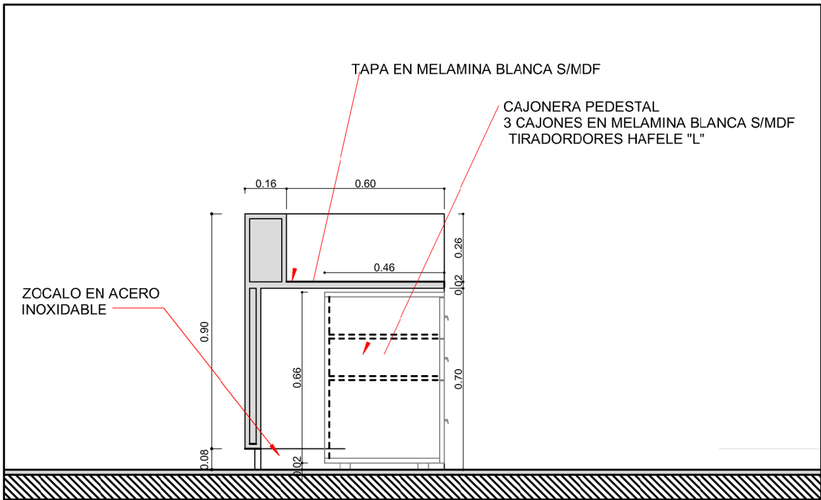
CORTE TRANSVERSAL
