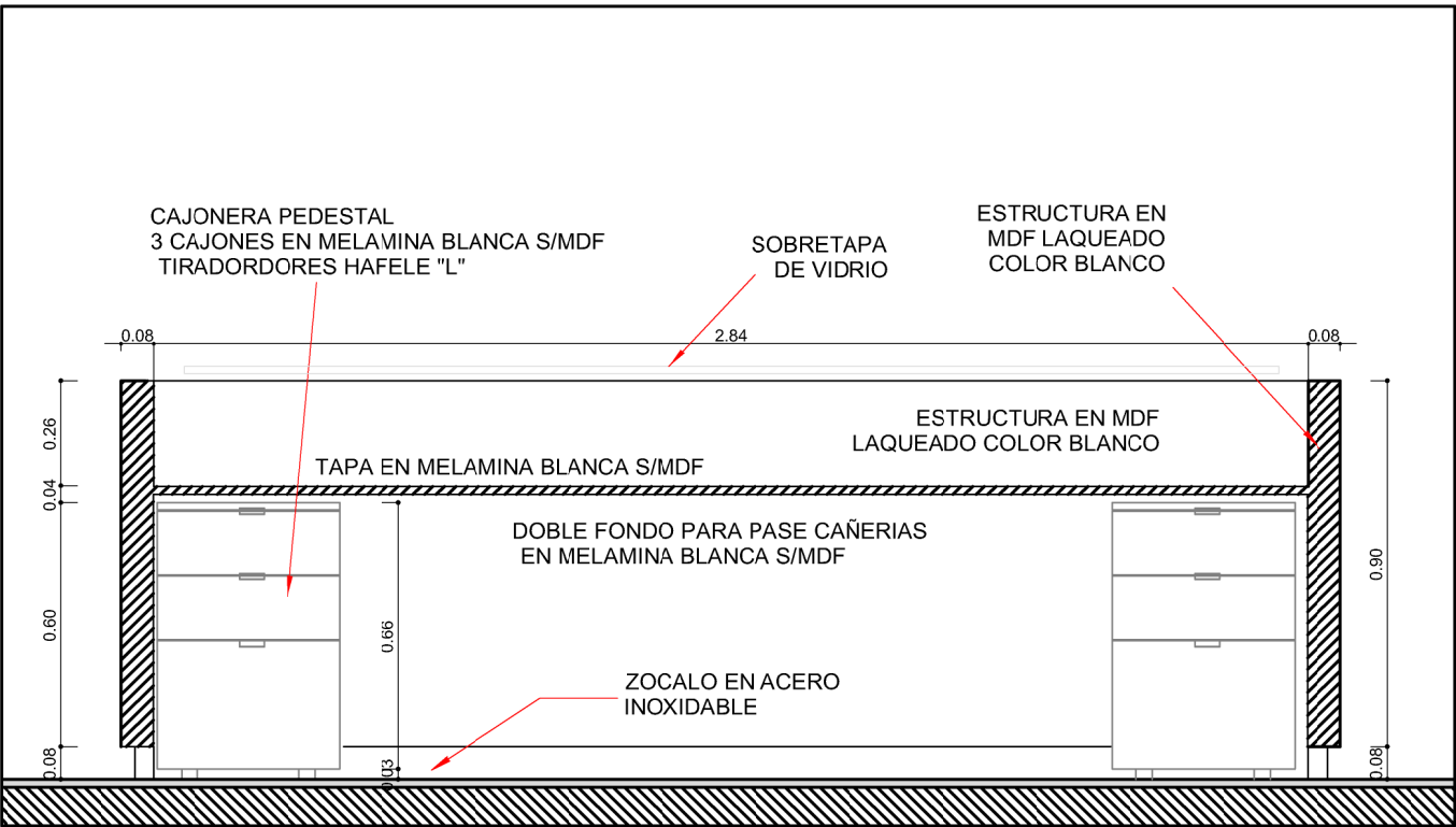
CORTE LONGITUDINAL
