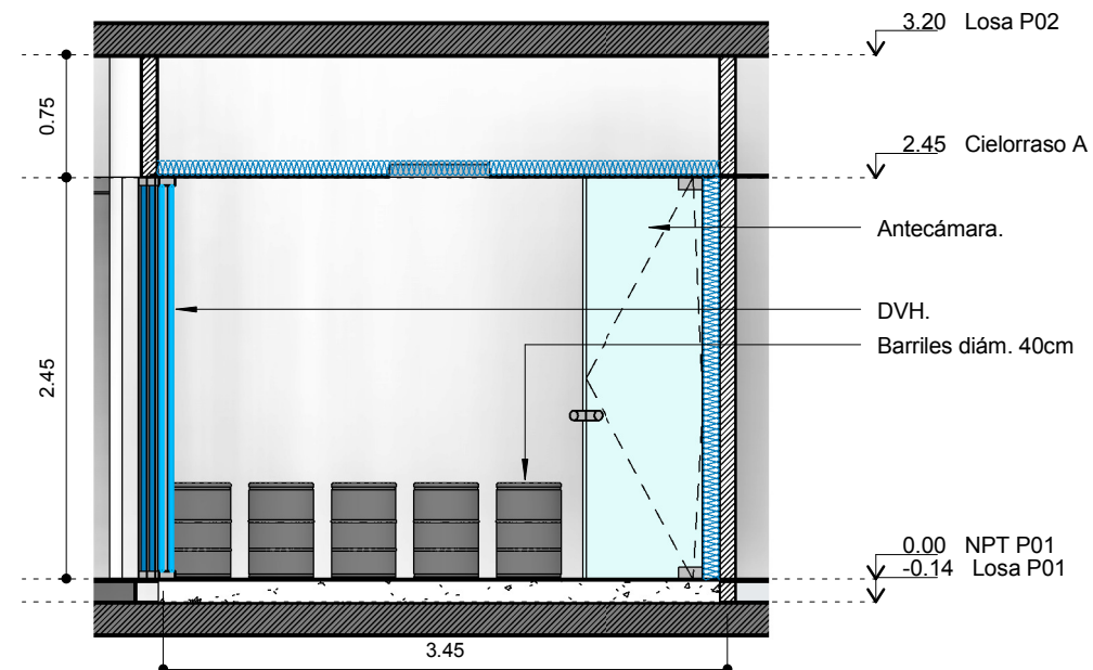
CORTE A
