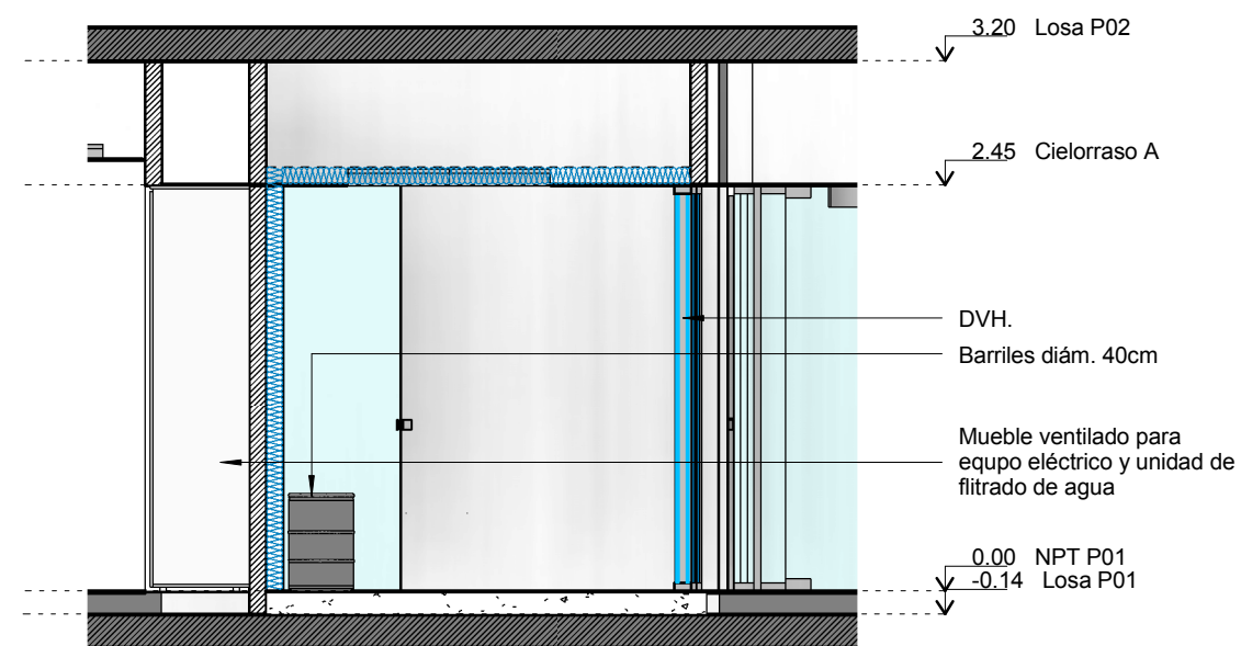
CORTE C
