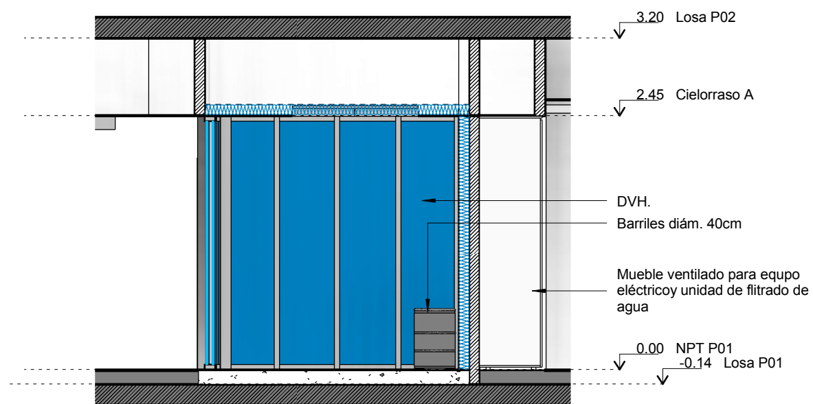
CORTE B
