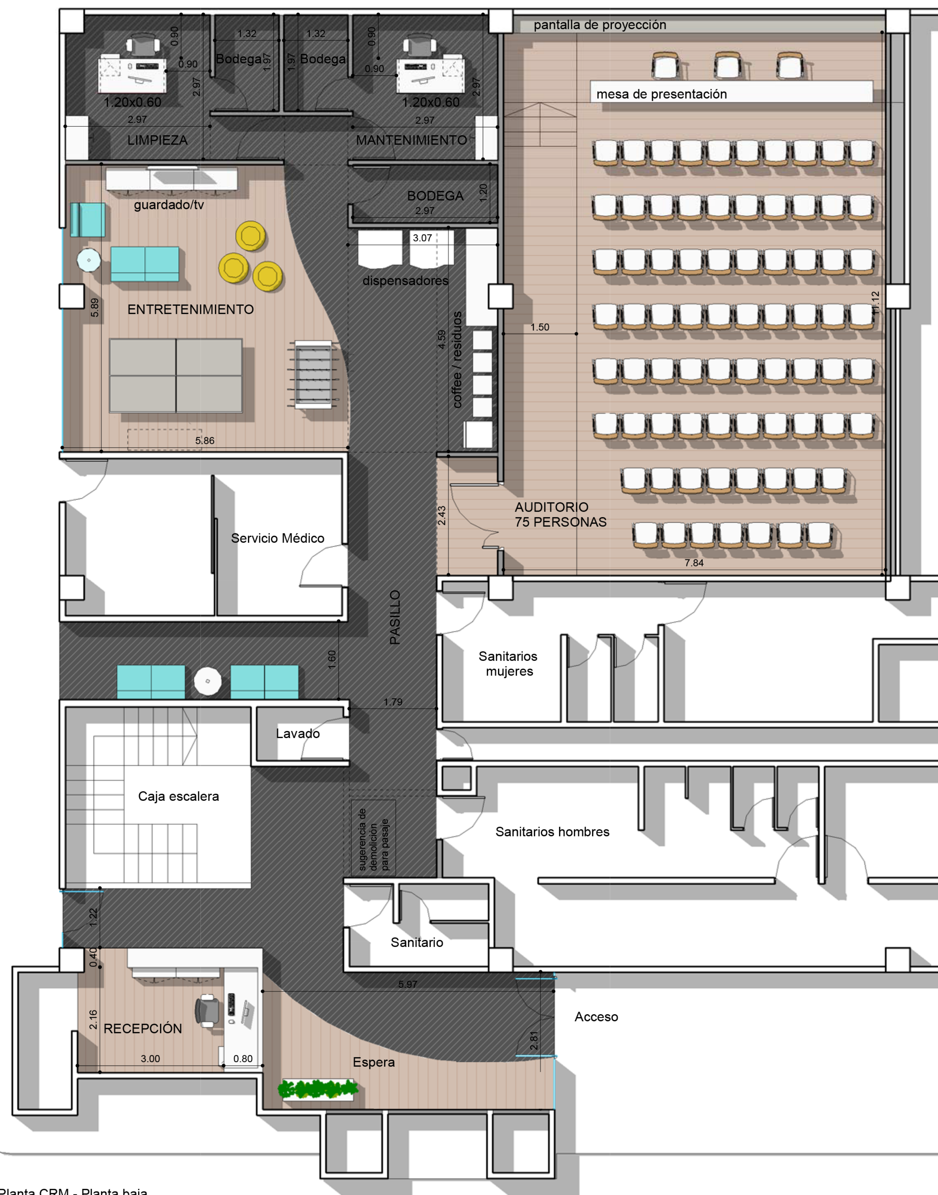
Planta CRM - Planta baja esc 1:100
