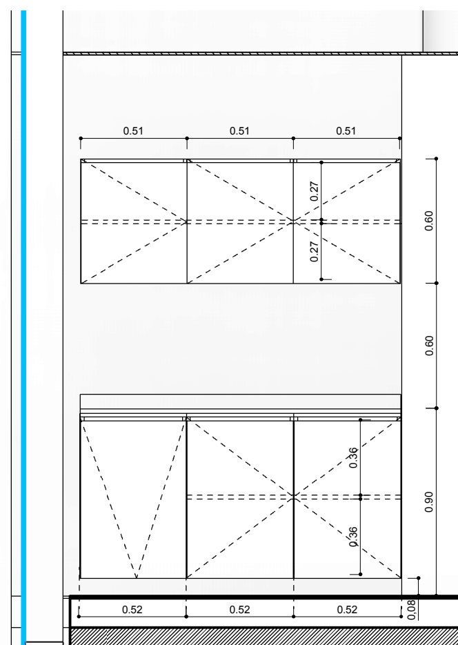
CORTE CP6
