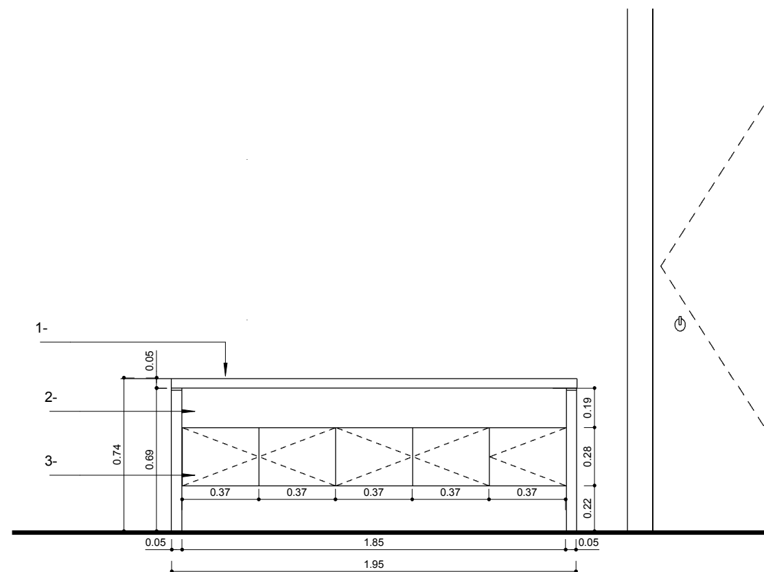
CORTE CN2
