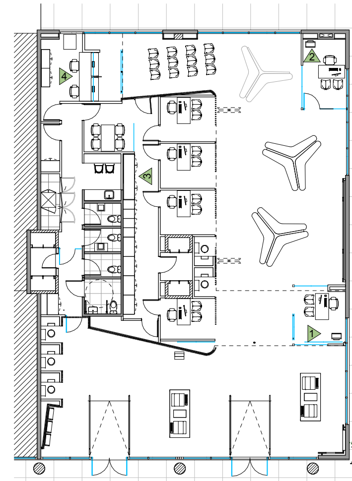
PLANTA UBICACION IMPRESORA SEGUN LAYOUT EQUIPAMINETO
