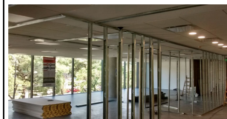
Piso 2- Acopio de placas. Armado de estructura de piso a cielorraso
