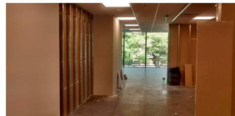
Piso 2- Colocacion de placas con espacio para buña Z
