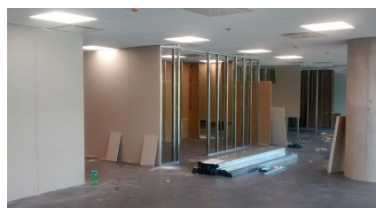
Piso 2- Armado de estructura.
