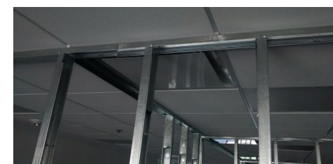
Piso 2- Acopio de placas. Armado de estructura de piso a cielorraso
