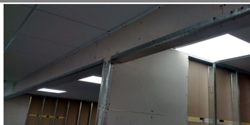
Piso 2- Emplacado de dinteles
