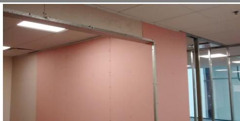
Piso 3- Ingreso de material para estructura de tabiques
