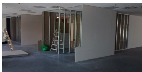
Piso 2- Placas de tabique 1 cara
