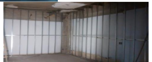
Canalizaciones para Iluminacion sobre cielorraso. Estructura para revestimiento de paredes. Subsuelo.
