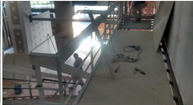
Colocacion de placas cementicias sobre nueva pasarela.
