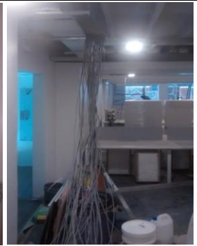
Instalación de tablero general pre-armado. Cableado de UTP por bandeja troncal.
