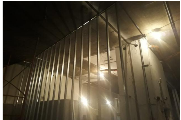
Inicios en estructura de tabique de Durlock
