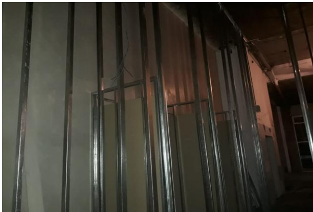
Estructura de tabique de Durlock
