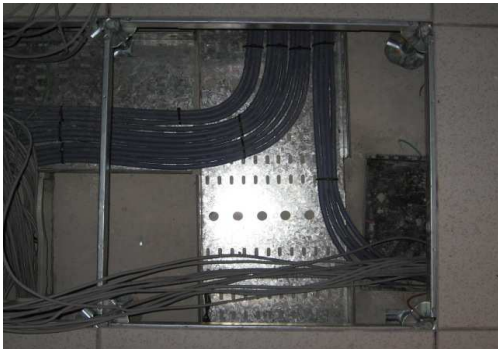
EJECUCIÓN DE CABLEADO BAJO PISO TÉCNICO EN DATA CENTER
