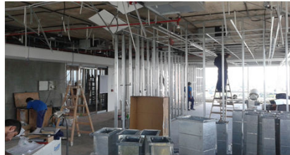
Ejecucion de Estructura de tabiquería de Placa roca de yeso
