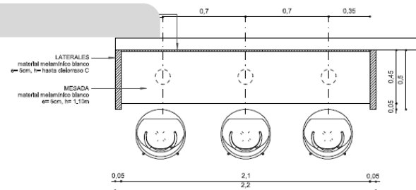
Me2 - Planta 1:20
