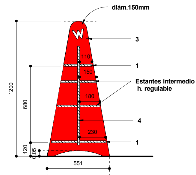
CORTE A
