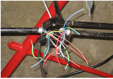
RECABLEADO DE INSTALACION ELECTRICA SOBRE CIELORRASOS SEGUN NORMATIVAS VIGENTES
