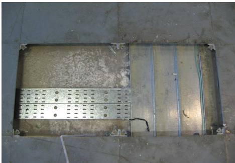
TENDIDO DE NUEVAS BANDEJAS BAJO PISO TECNICO
