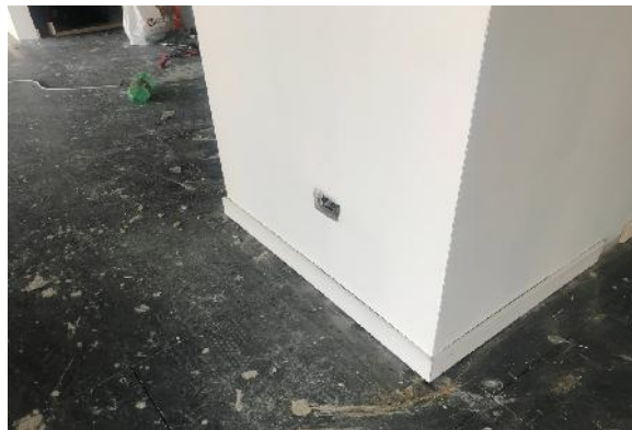
PREPARACION DE TABIQUES + COLOCACION DE ZOCALOS
